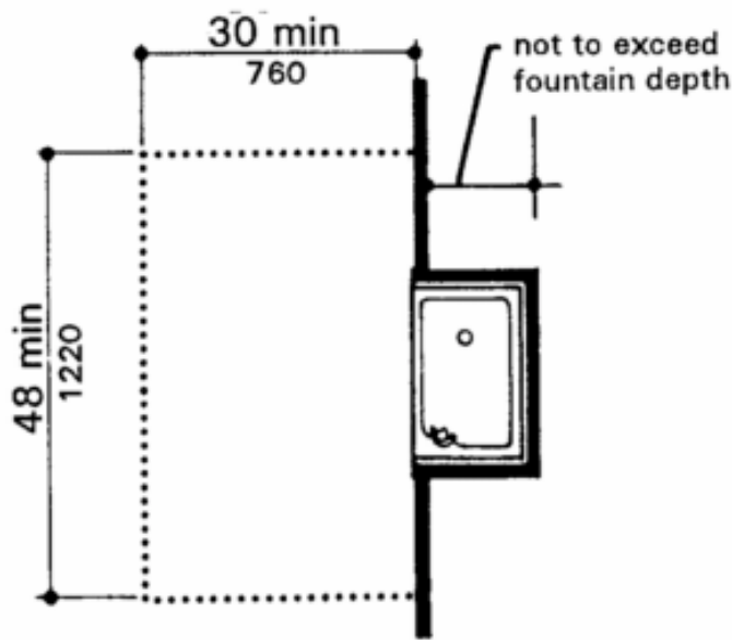
(d) Built-in Fountain or Cooler
